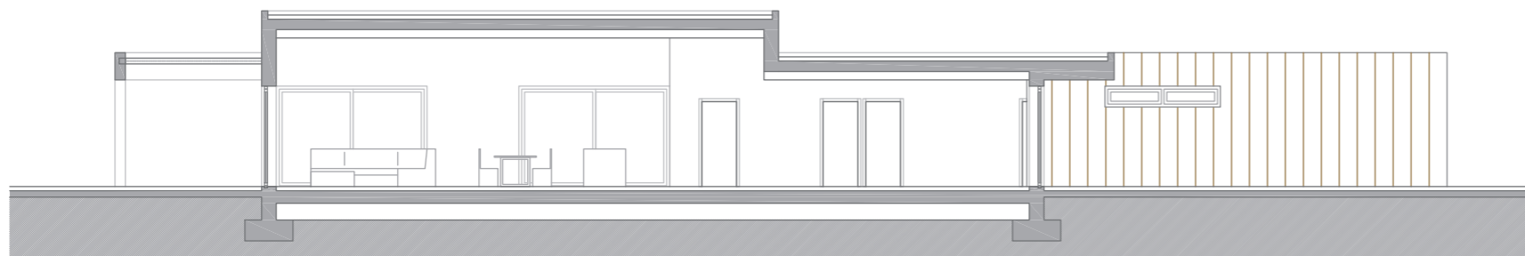
SECCIÓN C
