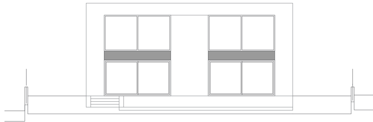
ALZADO SUR
