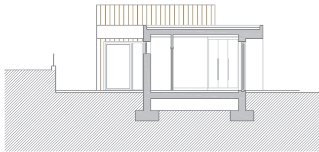
SECCIÓN A
