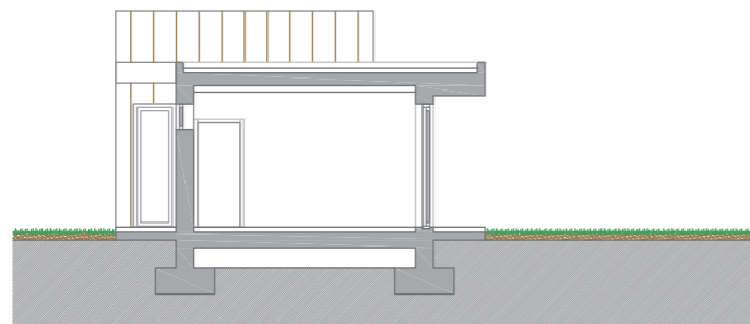
SECCIÓN A
