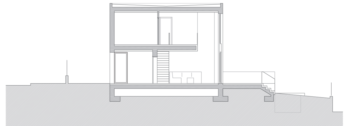
SECCIÓN A
