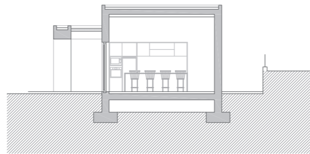
SECCIÓN B
